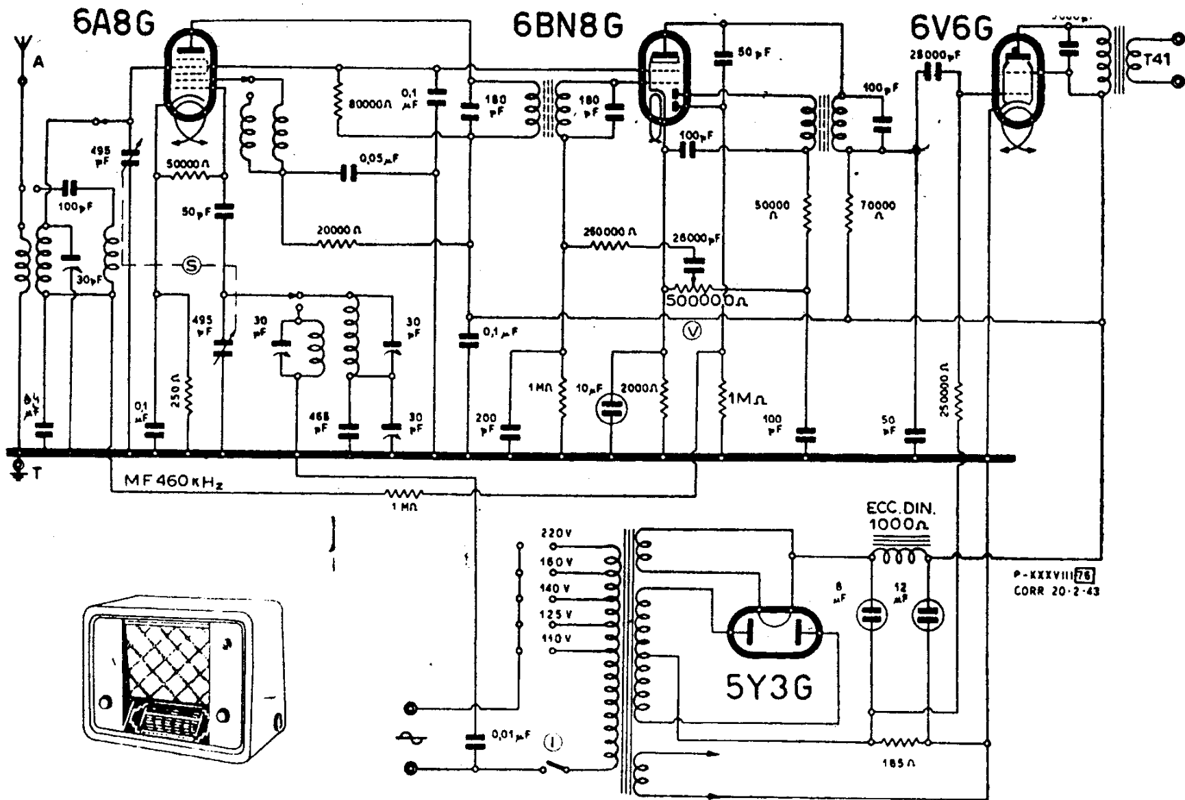
· WATT RADIO - MOD. « GEMMA »
